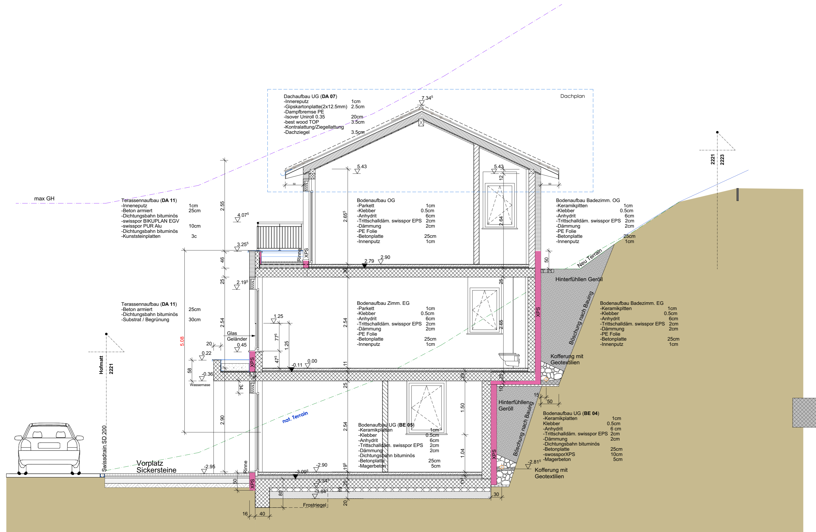
SCHNITT B_B
